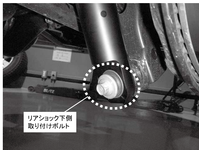
リアショック下側取り付けボルト
