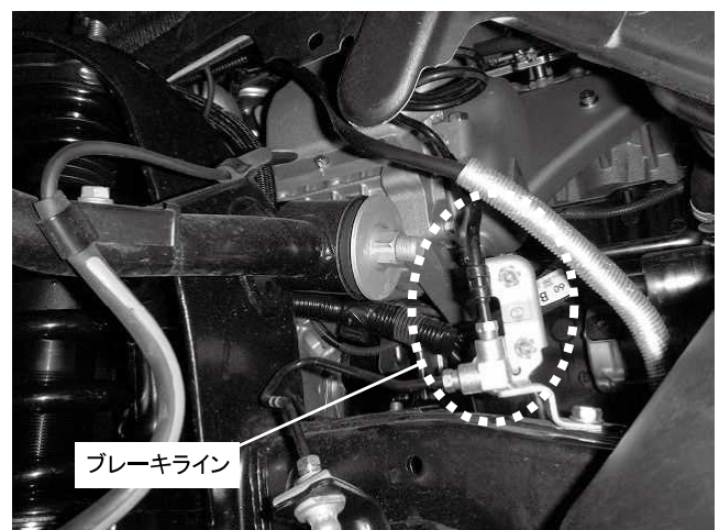
ブレーキライン フロントサスペンションアッパーアームの ボルト・ナットを締め付ける際、 ブレーキラインの破損に注意してください
