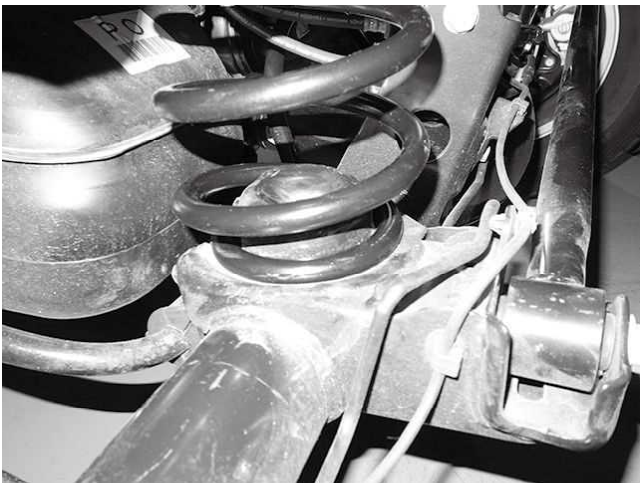
リアスプリングロア側取り付け状態 ※スプリングと車軸側の切り欠き位置が あっているか確認してください
