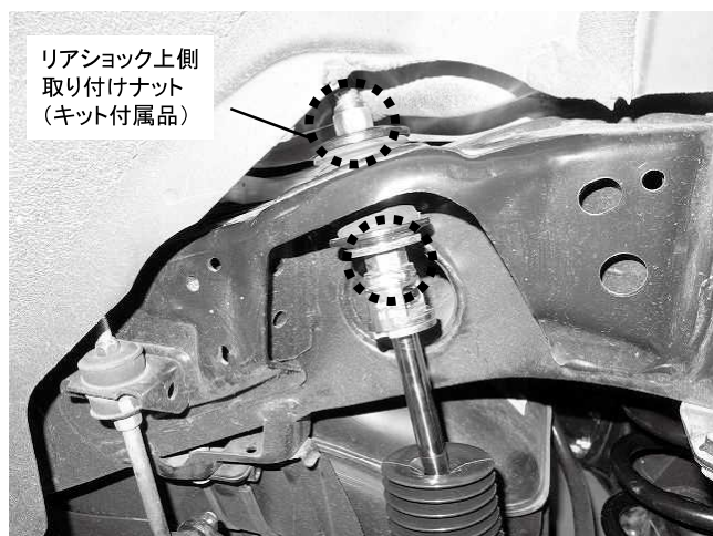
リアショック上側取り付けナット
