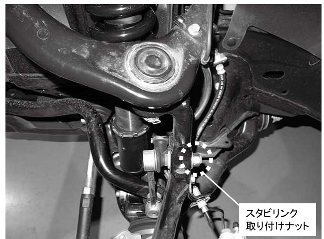
スタビリンク 取り付けナット 1カ所締め付け 締め付けトルク: 70\text{N}\cdot\text{m} ( 7.1\text{kgf}\cdot\text{m} )
