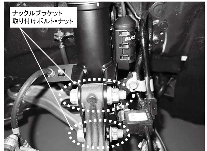
ナックルブラケット 取り付けボルト・ナット 2カ所締め付け 締め付けトルク: 155N・m (15.8kgf・m) ※ワッシャーも純正同様にに取り付けてください
