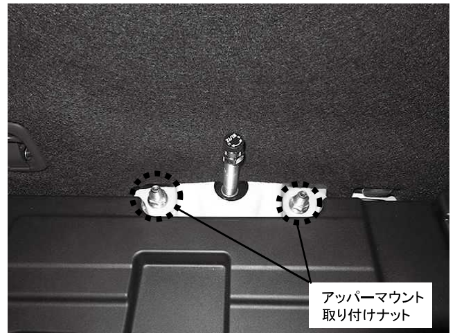
アッパーマウント取り付けナット 2カ所締め付け 締め付けトルク: 30N・m (3.1kgf・m) ※製品付属のM10ナットを使用してください
