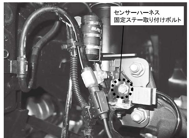
センサーハーネス固定ステー取り付けボルト 1カ所締め付け 締め付けトルク: 33N・m (3.4kgf・m)
