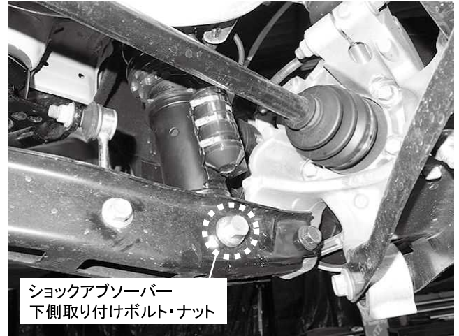
ショックアブソーバー下側取り付けボルト・ナット 1カ所締め付け 締め付けトルク: 85N・m (8.7kgf・m)
