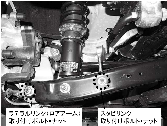
ラテラルリンク(ロアアーム)取り付けボルト・ナット 1カ所締め付け 締め付けトルク: 82.5N・m (8.4kgf・m) スタビリンク取り付けボルト・ナット
