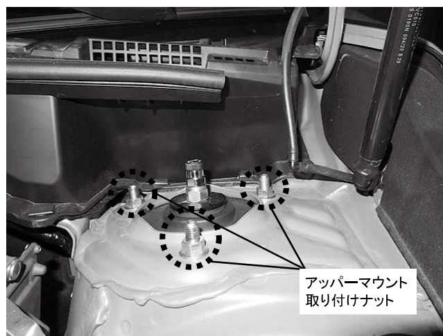
アッパーマウント取り付けナット 3カ所締め付け 締め付けトルク: 32\text{N}\cdot\text{m} ( 3.3\text{kgf}\cdot\text{m} ) ※製品付属のM10ナットを使用してください
