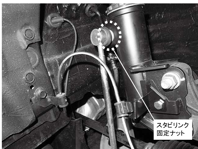
スタビリンク固定ナット 1カ所締め付け 締め付けトルク: 60\text{N}\cdot\text{m} ( 6.1\text{kgf}\cdot\text{m} )
