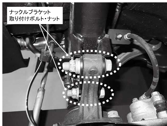
ナックルブラケット 取り付けボルト・ナット 2カ所締め付け 締め付けトルク: 155\text{N}\cdot\text{m} ( 15.8\text{kgf}\cdot\text{m} ) ※ワッシャーも純正同様に取付けてください
