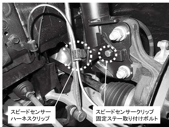
スピードセンサー ハーネスクリップ スピードセンサークリップ 固定ステー取り付けボルト 1カ所締め付け 締め付けトルク: 24\text{N}\cdot\text{m} ( 2.4\text{kgf}\cdot\text{m} ) スピードセンサーハーネスクリップ取り付け
