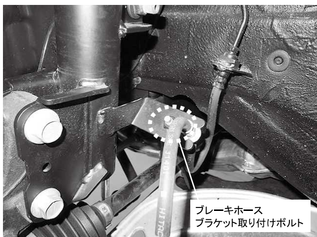
ブレーキホースブラケット取り付けボルト 1カ所締め付け 締め付けトルク: 33\text{N}\cdot\text{m} ( 3.4\text{kgf}\cdot\text{m} )
