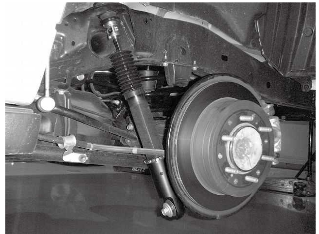
リアショック取り付け状態
