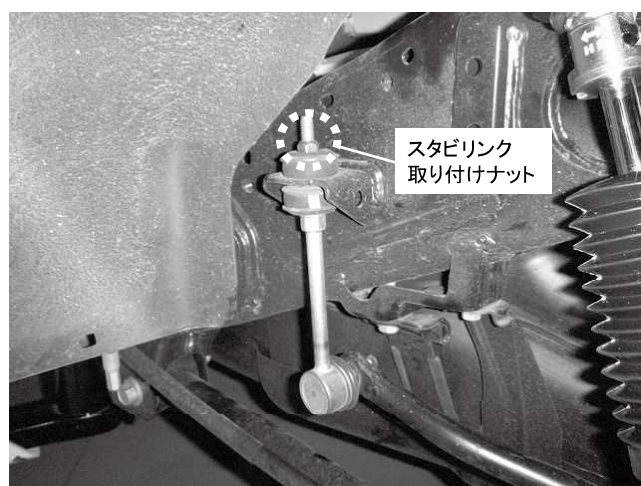
スタビリンク取り付けナット 1カ所締め付け 締め付けトルク: 15N・m(1.5kgf・m)
