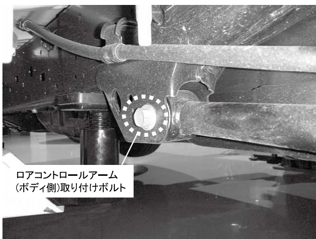
ロアコントロールアーム(ボディ側)取り付けボルト 1カ所締め付け 締め付けトルク: 130N・m(13.3kgf・m) ※アクスルビームをジャッキで支えながら取り付けし、 締め付けの際はしっかり車重をかけて締め付けてください
