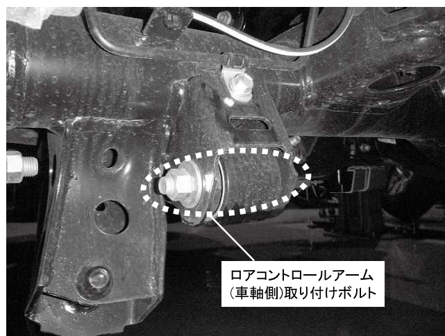
ロアコントロールアーム(車軸側)取り付けボルト・ナット 1カ所締め付け 締め付けトルク: 130N・m(13.3kgf・m) ※アクスルビームをジャッキで支えながら取り付けし、 締め付けの際はしっかり車重をかけて締め付けてください
