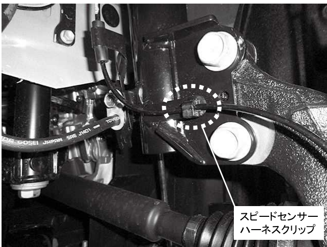
スピードセンサーハーネスクリップ取り付け ※クリップがブラケットに固定できない、またはハーネスが 突っ張ってしまう場合にはクリップをハーネスから取り外し、 クリップをロアブラケットに付けてからハーネスを取り付けてください
