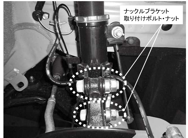
ナックルブラケット取り付けボルト・ナット 2カ所締め付け 締め付けトルク: 270N・m(27.5kgf・m)
