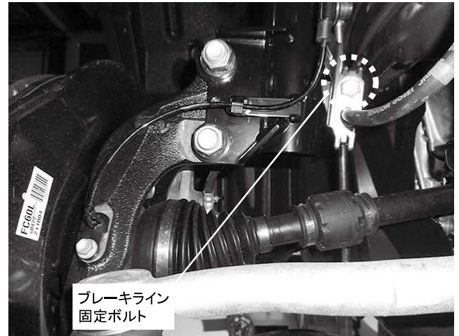
ブレーキライン固定ボルト 1カ所締め付け 締め付けトルク: 29N・m(2.9kgf・m) ※ネジ部に塗装がついて締め付けが渋い場合があります
