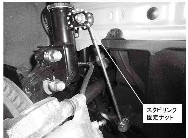
スタビリンク固定ナット 1カ所締め付け 締め付けトルク: 74N・m(7.5kgf・m) ※スタビリンクは純正品を使用してください
