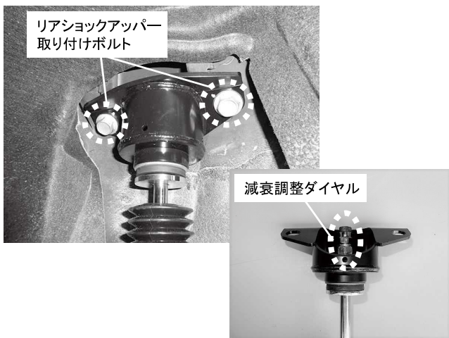
リアショックアッパース取り付けボルト 2カ所締め付け 締め付けトルク: 55\text{N}\cdot\text{m} ( 5.6\text{kgf}\cdot\text{m} ) ※減衰調整ダイヤルは構造上 アッパーマウント内部についています ※キット付属ダイヤルキャップを取り付けてください
