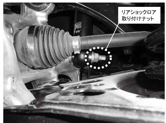
リアショックロア取り付けナット 1カ所締め付け 締め付けトルク: 125\text{N}\cdot\text{m} ( 12.7\text{kgf}\cdot\text{m} )
