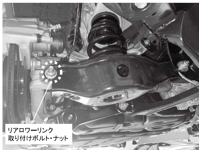
リアローリンク取り付けボルト・ナット 1カ所締め付け 締め付けトルク: 187.5N・m(19.0kgf・m)
