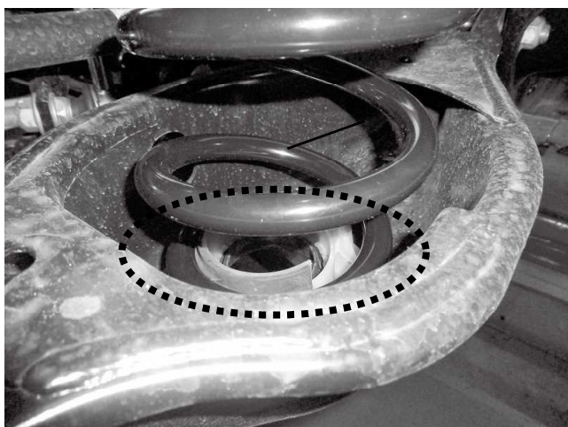
スプリングロアラバーがしっかりはまっているか確認してください また、スプリングの切り欠きの位置があっているかも確認してください
