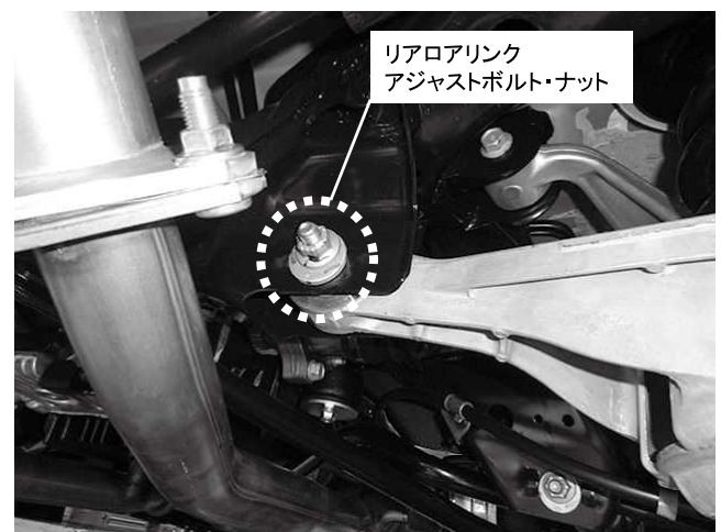
リアロアリンクアジャストボルト・ナット 1カ所締め付け 締め付けトルク: 72.5N・m(7.4kgf・m)
