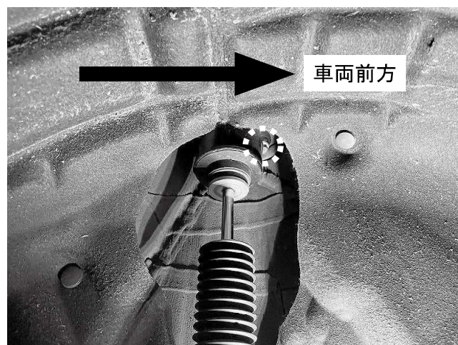
右(運転席)側リアショック取り付け状態 矢印の方向が車両前方側を示しています カラーは前方側のみに必ず取り付けください
