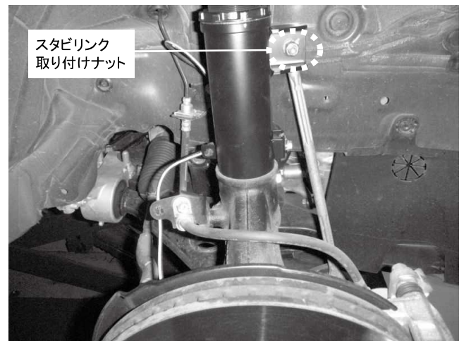
スタビリンク取り付けナット 1カ所締め付け 締め付けトルク: 64N・m (6.5kgf・m) ※スタビリンクは純正品を使用してください
