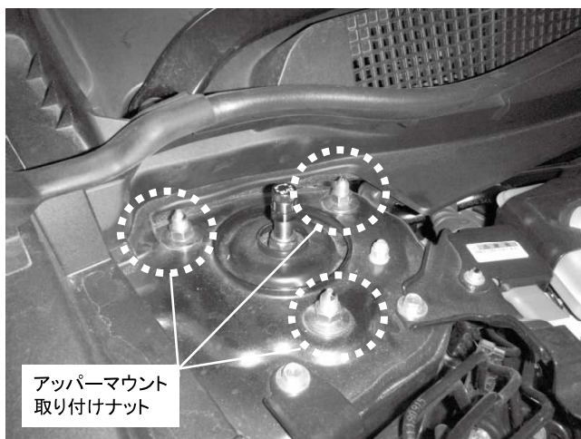
アッパーマウント取り付けナット 3カ所締め付け 締め付けトルク: 75N・m (7.6kgf・m) ※ナットは純正品を使用してください
