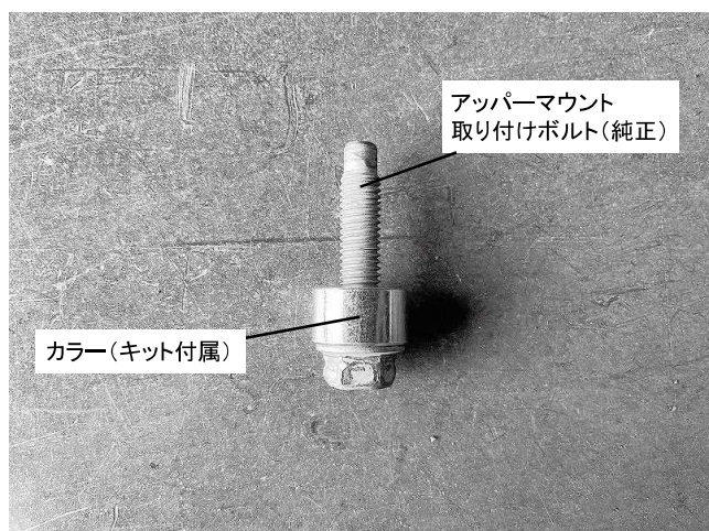
リアショックアッパーマウントを取り付ける際、 必ずキット付属のカラーを車両前方側のボルト のみに取り付けから、車両へ取り付けください
