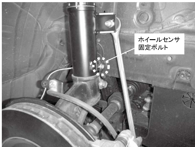
ホイールセンサ固定ボルト 1カ所締め付け 締め付けトルク: 9.5N・m (0.9kgf・m)
