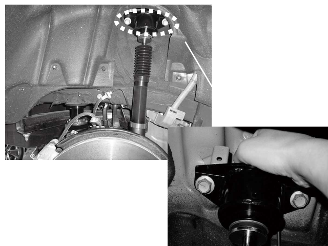
必要に応じて、タイヤハウス内のクリップを外し、 インナーフェンダーをめくると、リアショック上部に アクセスでき、減衰調整ダイヤルを回すことが可能です ダイヤルキャップを取り付けた状態で回すことができます
