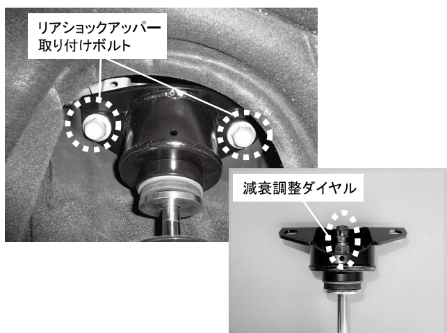
リアショックアッパー取り付けボルト 2カ所締め付け 締め付けトルク: 55\text{N}\cdot\text{m} ( 5.6\text{kgf}\cdot\text{m} ) ※減衰調整ダイヤルは構造上 アッパーマウント内部についています ※キット付属ダイヤルキャップを取り付けてください
