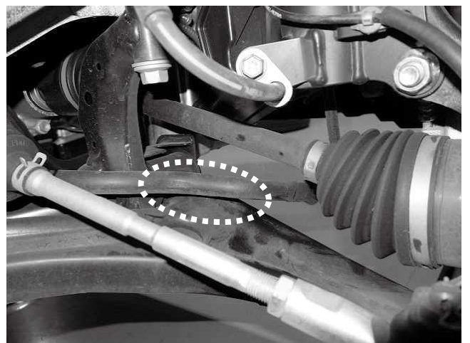
フロント右(運転席)側の取り付け後の写真になります ロアアームとスタビライザーが干渉していないか 確認してください ※写真は基準車高(寸法)の0G時状態です
