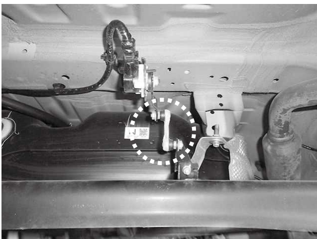
ヘッドランプオートレベリング機構付き車の場合 スプリング脱着時や車高調整の際には 取り付け向きや破損に注意してください
