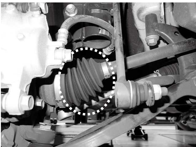
フロント右(運転席)アウト側のドライブシャフトとブーツの状態になります ※車高調整の際は、ドライブシャフトの傾きに注意してください ※リフトアップすることでドライブシャフトブーツに通常よりも多く負担がかかりますので、破損していないか定期的に確認を行ってください ※写真は基準車高(寸法)の0G時状態です
