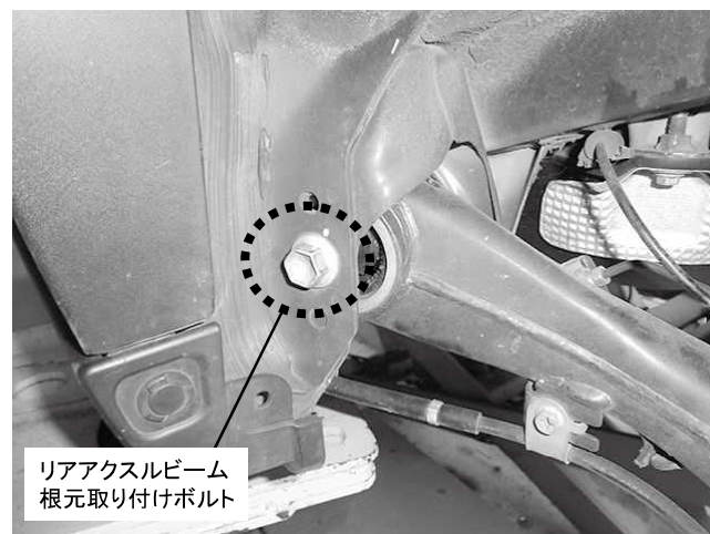
リアアクスルビーム根本取り付けボルト
