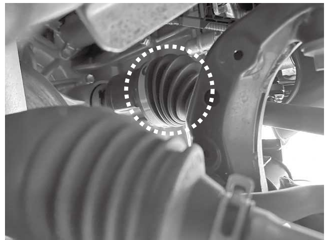
フロント右(運転席)イン側のドライブシャフトとブーツの状態になります ※車高調整の際は、ドライブシャフトの傾きに注意してください ※リフトアップすることでドライブシャフトブーツに通常よりも多く負担がかかりますので、破損していないか定期的に確認を行ってください ※写真は基準車高(寸法)の0G時状態です
