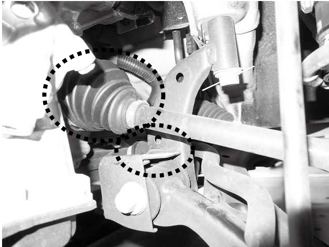
フロント左(助手席)イン側のドライブシャフトとブーツの状態になります ※車高調整の際は、ドライブシャフトの傾きに注意してください ※ドライブシャフトとメンバーフレームが干渉していないか確認してください ※リフトアップすることでドライブシャフトブーツに通常よりも多く負担がかかりますので、破損していないか定期的に確認を行ってください ※写真は基準車高(寸法)の0G時状態です
