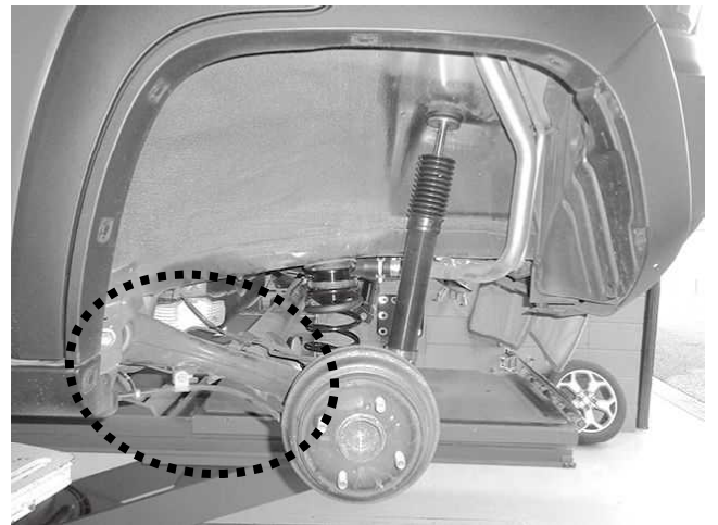
スプリングの脱着時や車高調整した際、 リアアクスルビーム根元のスピードセンサーハーネス の破損に注意してください またブレーキホースやハーネス類の 突っ張り状態を確認してください
