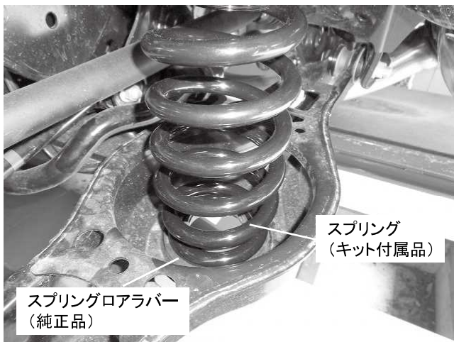
リアスプリング取り付け状態(下側) ※スプリングロアラバーがしっかりはまっているか 確認してください ※必要に応じてキット付属のスプリングチューブを使用してください
