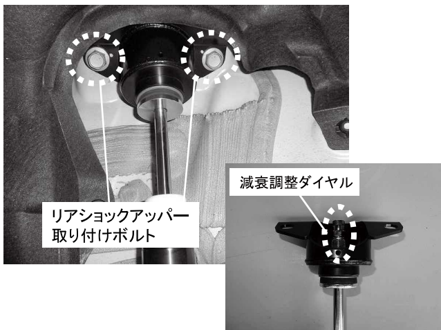
リアショックアッパー取り付けボルト 2カ所締め付け 締め付けトルク: 60\text{N}\cdot\text{m} ( 6.1\text{kgf}\cdot\text{m} )
