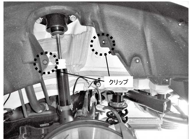
必要に応じて、タイヤハウス内のクリップを外し、インナーフェンダーをめくると、リアショック上部にアクセスでき、減衰調整ダイヤルを回すことが可能です
