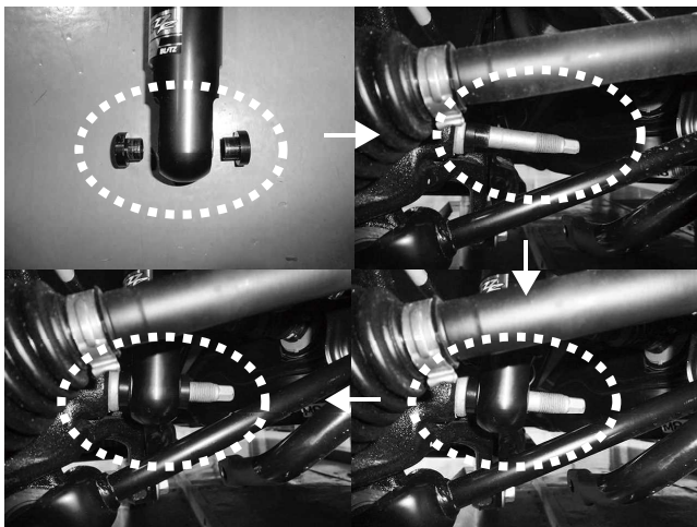
リアロアブラケット取り付けの際、そのままだとショックとボディが干渉取り付けにくい場合があります その際はロアブラケットからカラーを取り外して、「カラー⇒ブラケット⇒カラー」の順に入れていくと取り付けしやすいです
