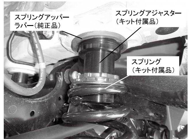
リアスプリング取り付け状態(上側) ※スプリングアッパーラバーがしっかりはまっているか 確認してください ※必要に応じてキット付属のスプリングチューブを使用してください
