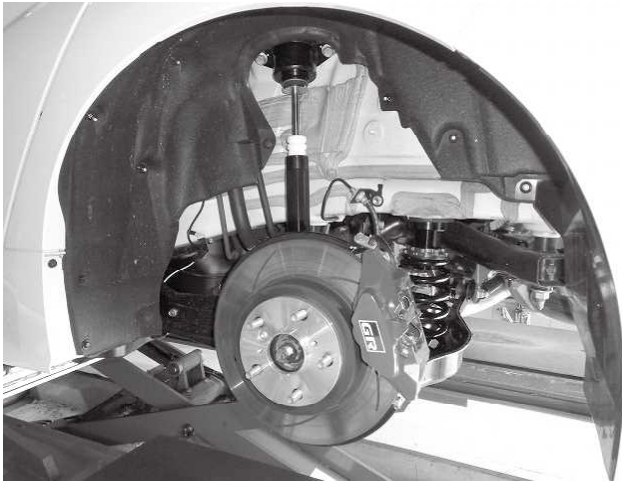
リア左側(助手席側)取り付け状態
