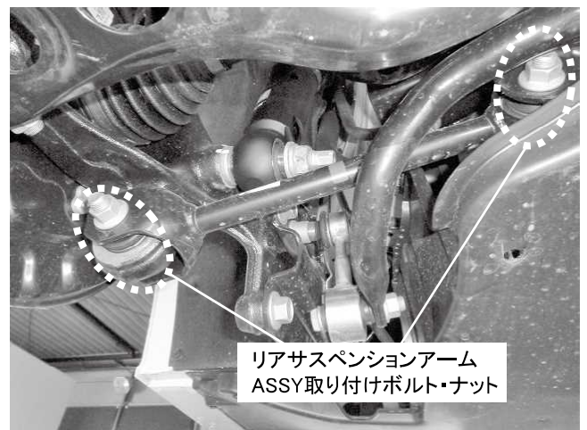
リアサスペンションアーム ASSY取り付けボルト・ナット 2カ所締め付け 締め付けトルク: 73N・m(7.4kgf・m) ※切り離さない場合でも一度緩めて1G状態で 締め直しをすることをお勧めいたします
