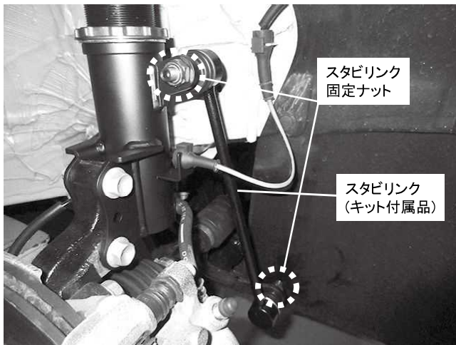
スタビリンク固定ナット 2カ所締め付け 締め付けトルク: 50N・m(5.0kgf・m) ※スタビリンクはキット付属品を使用してください
