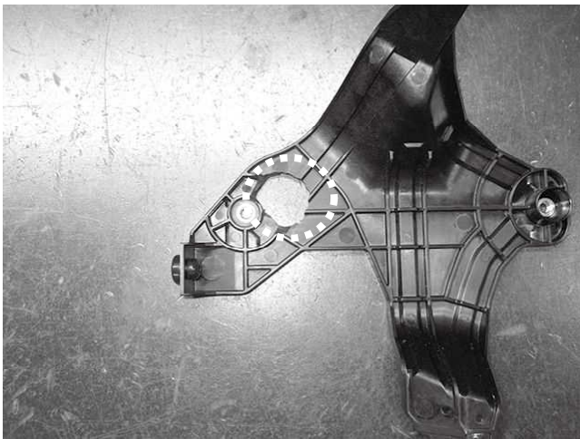
ECU固定ブラケット加工状態 左側(助手席側)のショック上部にECUがあり、 ECU固定ブラケットと減衰ダイヤルが干渉する 可能性があります その際は上写真のように加工をお願いします
