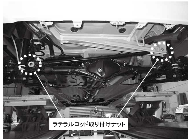
ラテラルロッド取り付けナット 2ヵ所締め付け 締め付けトルク: 65\text{N}\cdot\text{m} ( 6.7\text{kgf}\cdot\text{m} ) ※一度緩めて1G状態で再度締め直しすることをお勧めいたします
