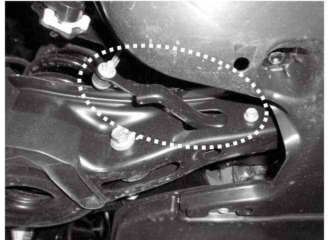
リアスプリング脱着時、ハイトコントロールセンサの破損に注意してください
