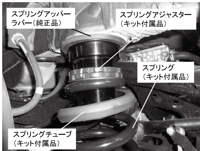
リアスプリング取り付け状態(上側)
