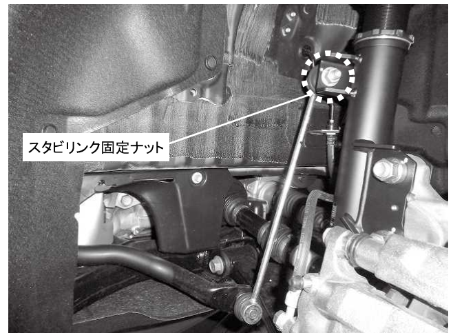
スタビリンク固定ナット スタビリンク固定ナット 2カ所締め付け 締め付けトルク: 74N・m (7.6kgf・m) ※スタビリンクは純正品を使用してください
