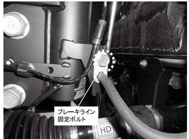
ブレーキライン 固定ボルト ブレーキライン固定ボルト 1カ所締め付け 締め付けトルク: 29N・m (3.0kgf・m) ※ネジ部に塗装がついて締め付けが渋い場合があります
