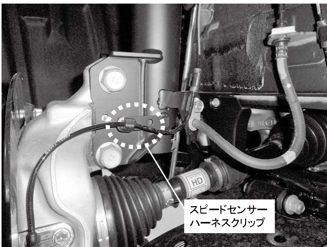
スピードセンサー ハーネスクリップ スピードセンサーハーネスクリップ取り付け ※クリップがブラケットに固定できない、またはハーネスが 突っ張ってしまう場合にはクリップをハーネスから取り外し、 クリップをロアブラケットに取り付けてからハーネスを取り付けて 調整を行ってください
