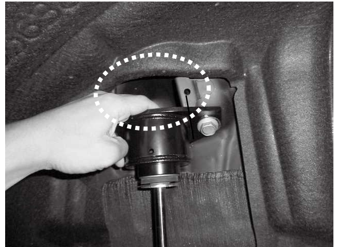
リアショック上部のスペースから、 減衰調整ダイヤルを回すことが可能です
