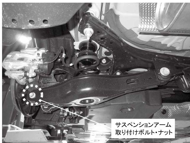
サスペンションアーム取り付けボルト・ナット 1カ所締め付け
