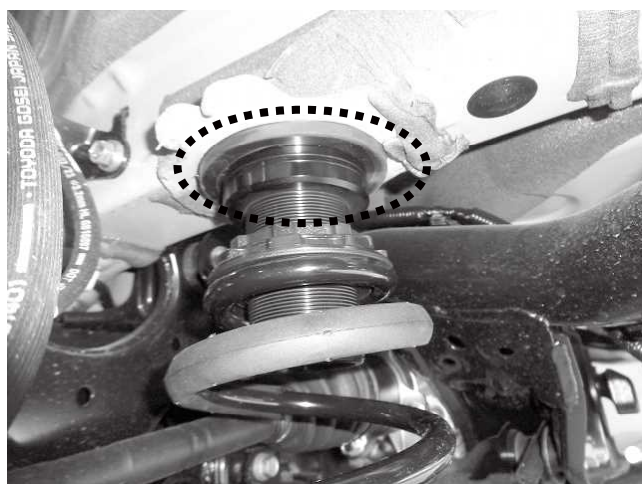
スプリングアッパーラバーがしっかりはまっているか 確認してください
