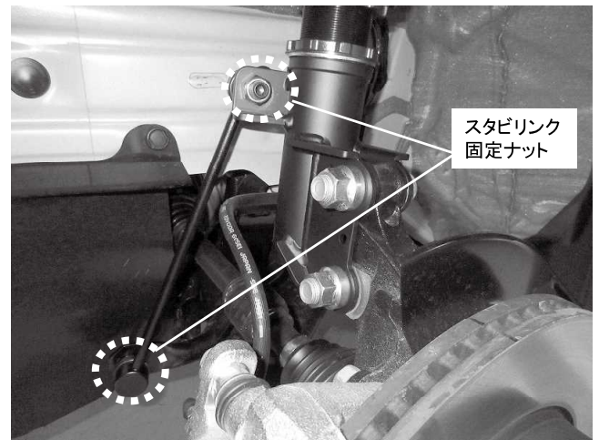
スタビリンク固定ナット 2カ所締め付け 締め付けトルク: 74N・m(7.5kgf・m) ※キット付属のスタビリンクを使用してください
