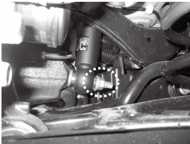
リアショックロア取り付けナット 1カ所締め付け
