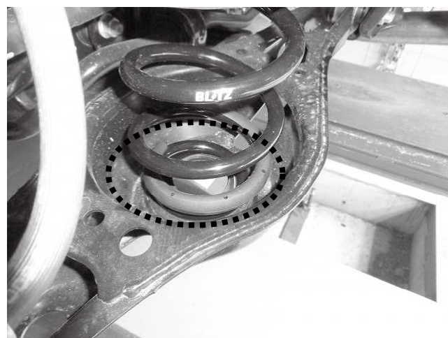
スプリングアロアラバーがしっかりはまっているか 確認してください
