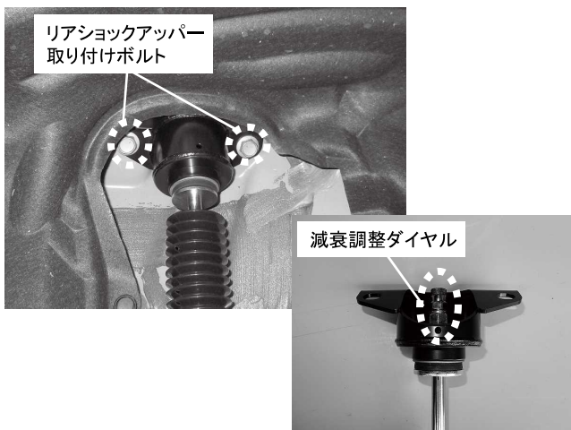
リアショックアッパース取り付けボルト 2カ所締め付け 締め付けトルク: 55N・m(5.6kgf・m)
