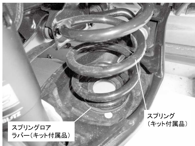
リアスプリング取り付け状態 (ロアアーム側)
