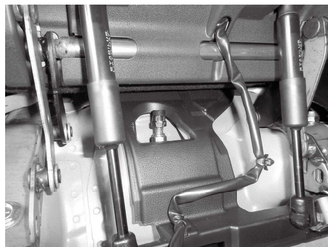
トップナット締め付け状態 ※写真はサードシート下部パネルを取り外した状態ですが、 キット取り付け後も左右ともに加工なしで サードシート下部パネルを取り付けが出来ます
