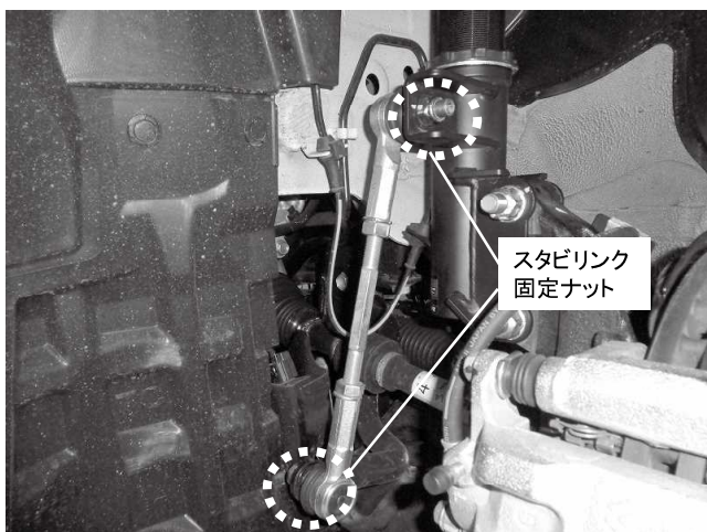
スタビリンク固定ナット 2カ所締め付け 締め付けトルク: 84N・m(8.6kgf・m) ※長さを調整しキット付属の スタビリンクを使用してください
