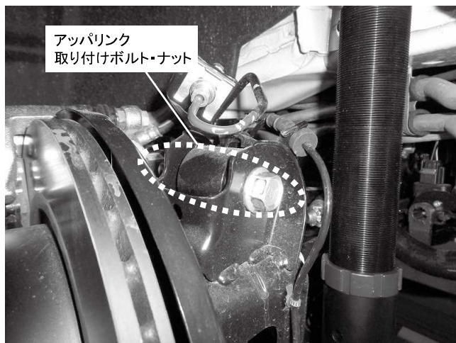
アッパリンク取り付けボルト・ナット 1カ所締め付け 締め付けトルク: 150\text{N}\cdot\text{m} ( 15.3\text{kgf}\cdot\text{m} ) ※一度緩めて1G状態で締め直しすることをお勧め致します
