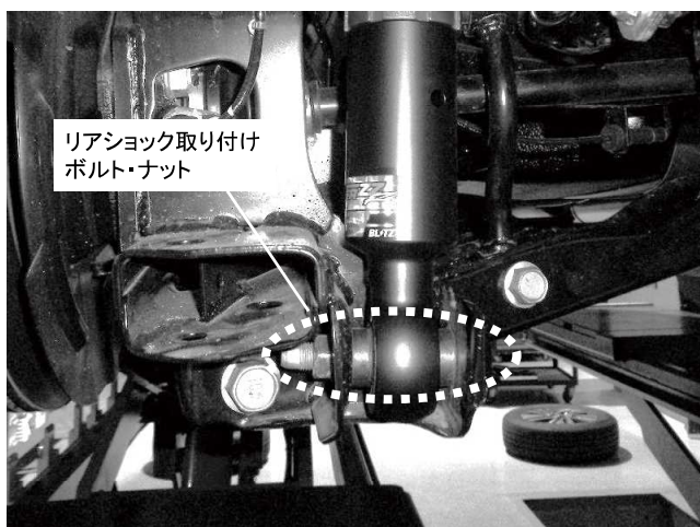
リアショック取り付けボルト・ナット 1カ所締め付け 締め付けトルク: 138\text{N}\cdot\text{m} ( 14.0\text{kgf}\cdot\text{m} )
