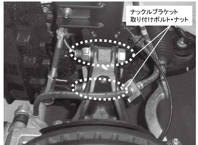
ナックルブラケット 取り付けボルト・ナット 2カ所締め付け 締め付けトルク: 142N・m(14.5kgf・m) ※ショックアブソーバーナックルブラケット上側取り付け穴は 長穴になっており、キャンバー調整が可能です 左右で位置を合わせて取り付けてください
