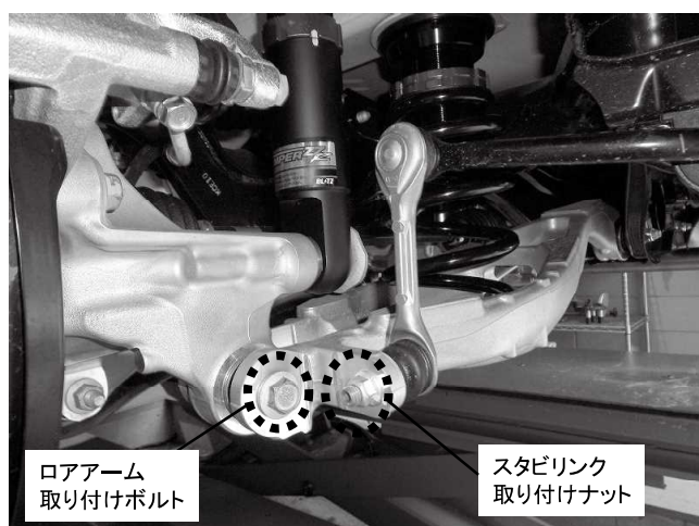
ロアアーム取り付けボルト 1カ所締め付け 締め付けトルク: 58\text{N}\cdot\text{m} ( 5.9\text{kgf}\cdot\text{m} ) スタビリンク取り付けナット 1カ所締め付け 締め付けトルク: 58\text{N}\cdot\text{m} ( 5.9\text{kgf}\cdot\text{m} )
