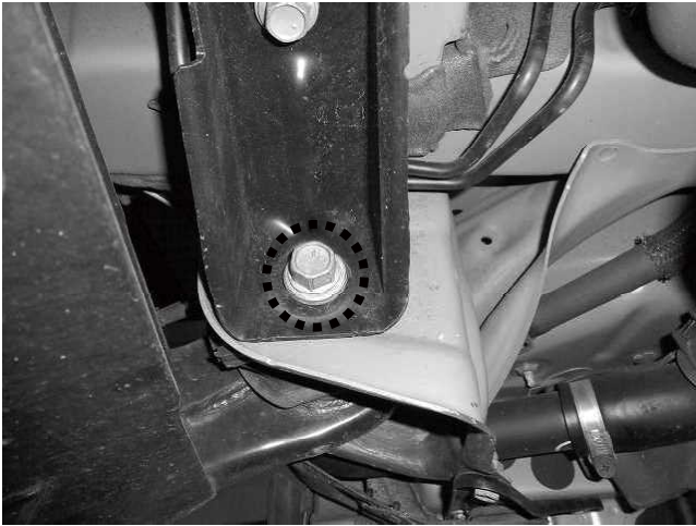
トーションビーム取り付けボルト 締め付けトルク: 110.5N・m(11.3kgf・m)
