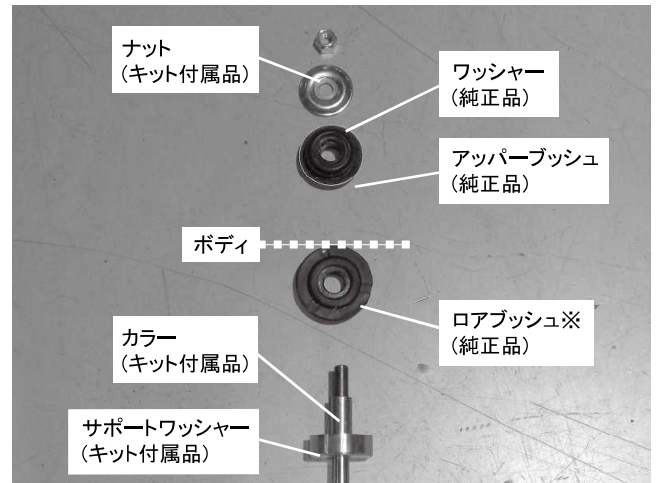
上写真を参照し、車両に取り付けてください トップナット締め付け 締め付けトルク: 30.6N・m(3.12kgf・m) ※下写真も参照して取り付けてください
