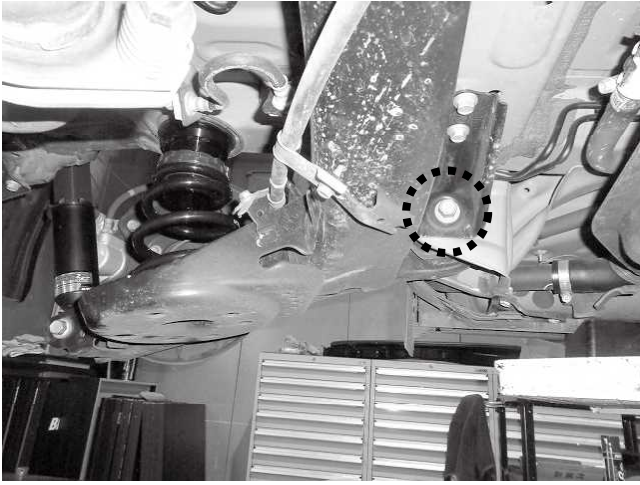
トーションビーム取り付けボルト 締め付けトルク: 110.5\text{N}\cdot\text{m} ( 11.3\text{kgf}\cdot\text{m} ) ※一度緩めて1G状態で締め直しすることをお勧め致します
