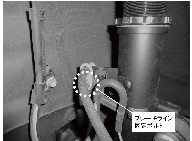
ブレーキライン固定ボルト 1カ所締め付け 締め付けトルク: 18.5N・m(1.9kgf・m) ※ネジ部に塗装がついて締め付けが渋い場合があります ※スピードセンサーハーネスと共締めしてあります
