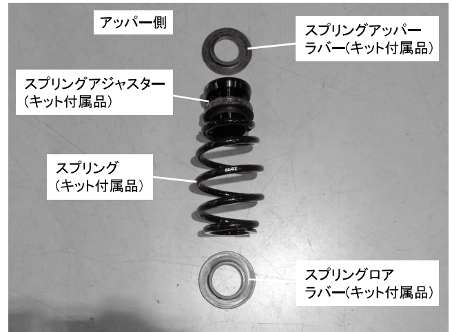
上写真を参照し、スプリングを車両に取り付けてください ※左下写真も参照してください
