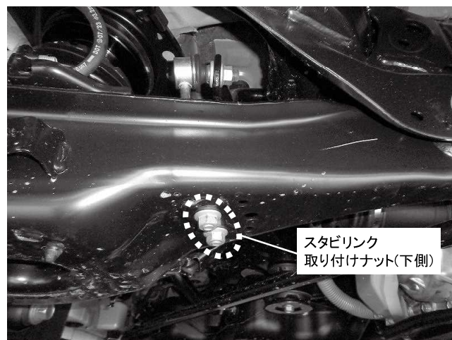
スタビリンク取り付けナット(下側)
