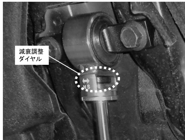
リアショックアブソーバー取り付け状態
