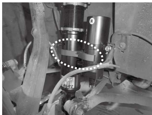
このキットのショックアブソーバーとリザーバータンクを 固定しているステーのボルトは1ヶ所のみになります。 しっかりと固定してください。
