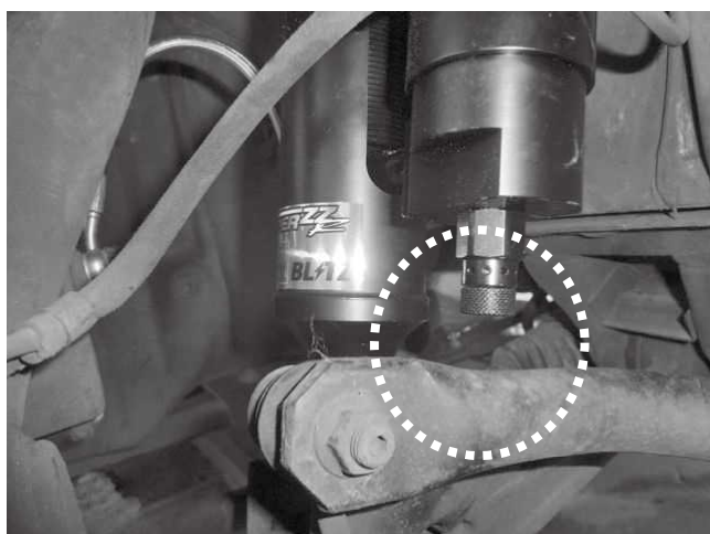
リザーバータンクとスタビライザーとの 干渉に注意してください。 ※車高を下げる場合特に注意してください。
