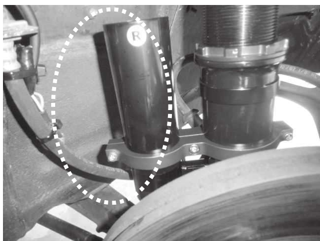
ステアリングをきった状態で、リザーバータンク (固定ステア)とインナーフェンダーとの干渉がないか 確認してください。
