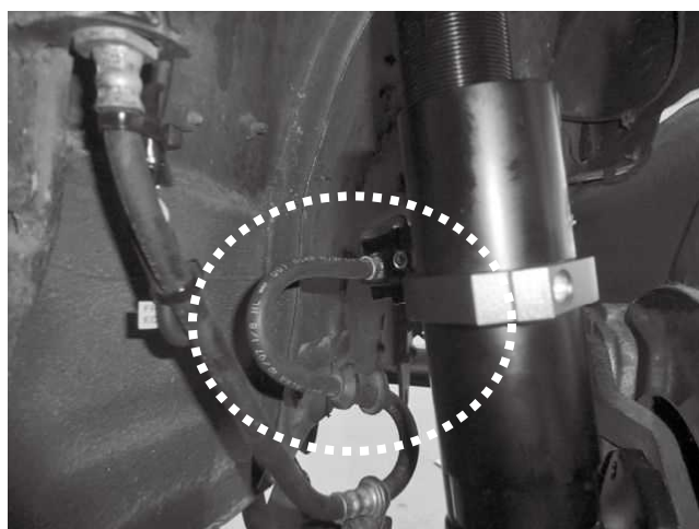
リザーバータンク(固定ステア)とブレーキラインとの 干渉に注意してください。 ※上写真は純正ブレーキラインではありません。
