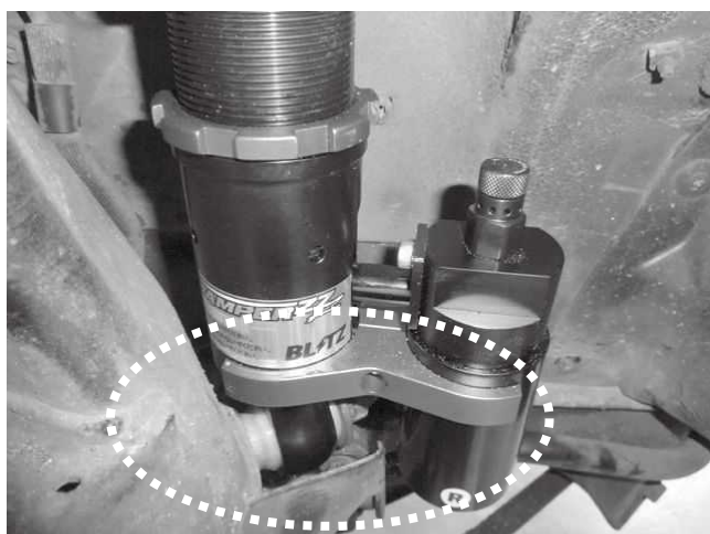
リザーバータンク(固定ステー)と ナックルなどとの干渉に注意してください。
