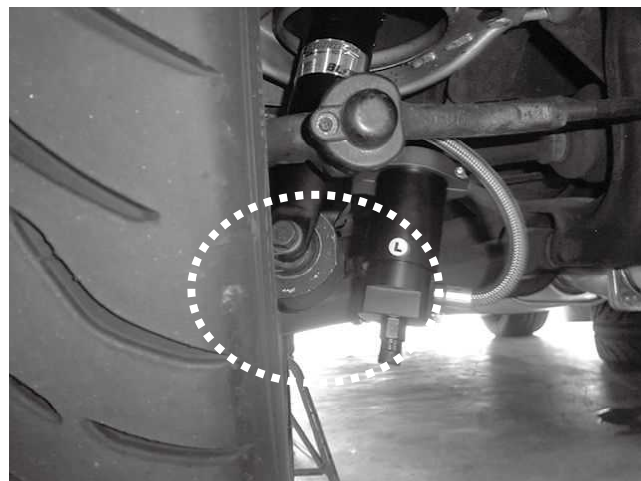
リア タイヤ・ホイールクリアランス 17×9.0J INSET20 255/40R17装着状態 ※取り付け後クリアランス確認をお願いします。
