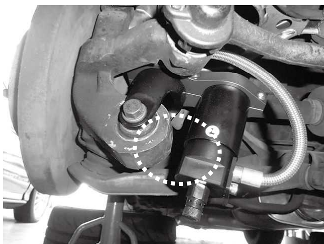
リザーバートankと ナックル取り付け部分との 干渉に注意してください。
