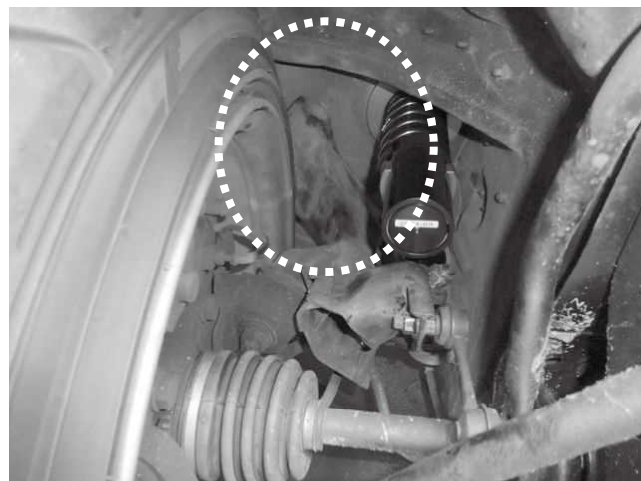
フロント タイヤ・ホイールクリアランス 17×9.0J INSET22 245/40R17装着状態 ※取り付け後クリアランス確認をお願いします。
