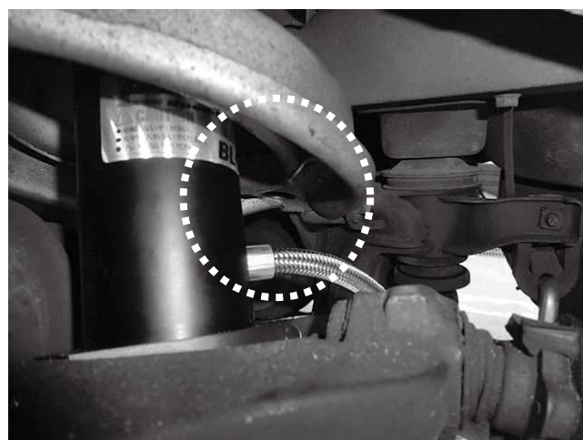
メッシュホースとアッパーアームとの 干渉に注意してください。 ※車高を上げる場合特に注意してください。 ※画像は基準車高時のフルバンプ状態です。
