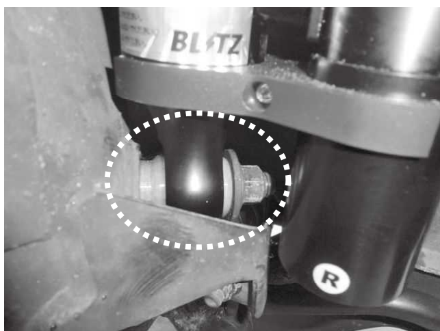
ロアブラケットの取り付けは長い方を ナックル側にして取り付けてください。 ※取り付けにくい場合はアッパーアームのボルトを 緩めるなどしてナックルを下げて作業を行ってください。
