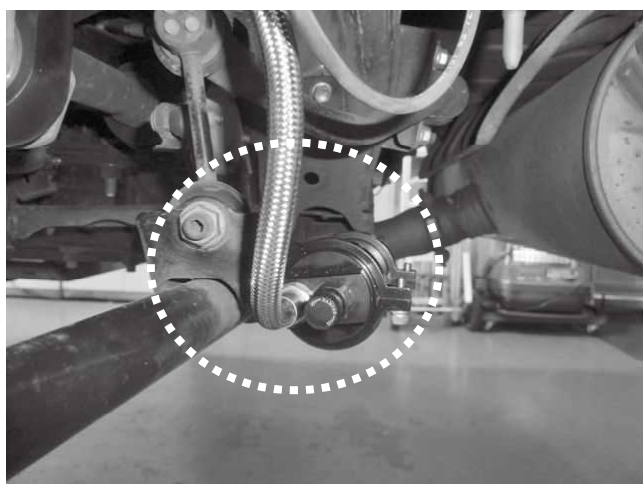
リザーバータンク・ホースと ロアアーム、スタビリンク取り付け位置との 干渉に注意してください。
