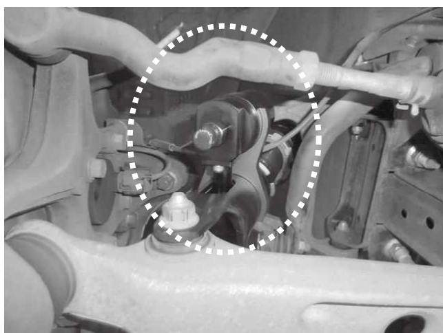
リザーバータンクと近接アームなどとの クリアランスに注意してください。
