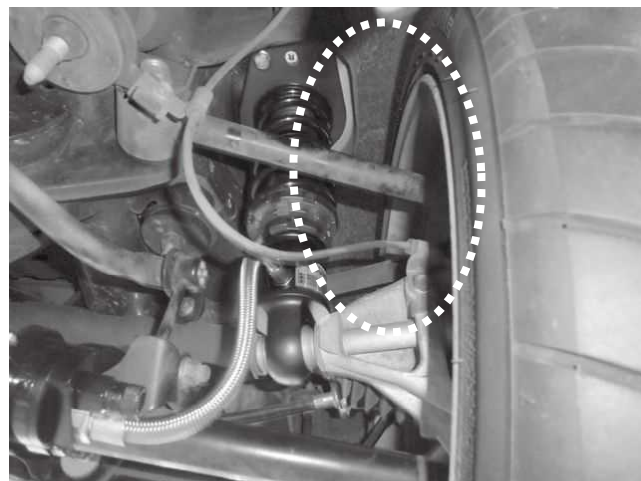
リア タイヤ・ホイールクリアランス 純正ホイール(18インチ)・タイヤ装着状態 ※取り付け後クリアランス確認をお願いします。
