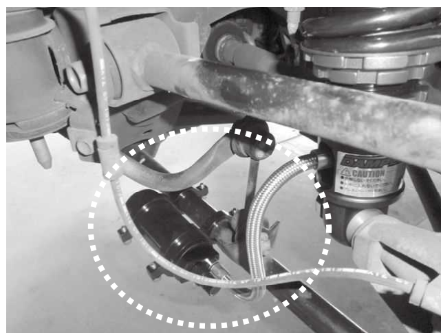
リザーバータンク・ホースと ロアアーム、スタビリンク、スピードセンサー ハーネスとの干渉に注意してください。
