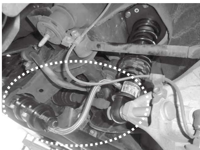
ロアアームに付属バンドを2個使用し 上写真のようにリザーバータンクを 固定してください。
