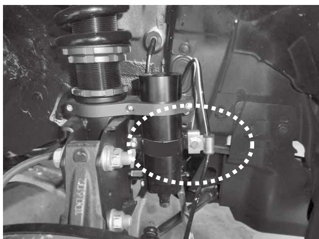
スピードセンサーラインはリザーバータンクに 付属バンドを使用し取り付けてください。
