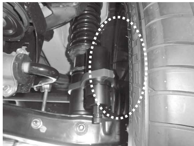
リア タイヤ・ホイールクリアランス 純正ホイール装着状態 ※取り付け後クリアランス確認をお願いします。
