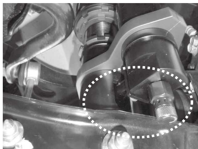
リザーバタンクとロアアームとの干渉に 注意してください。 ※車高を下げる場合特に注意してください。
