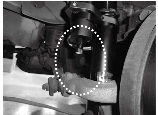
車高を下げる際、リザーバートankと ナックルとの干渉に注意してください。
