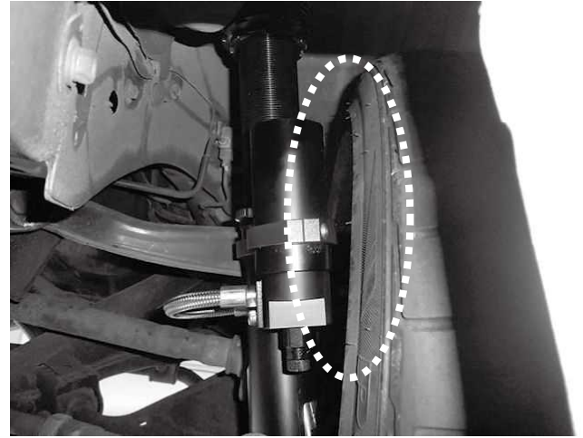
リア タイヤ・ホイールクリアランス 18×8.0J INSET35 235/40R18装着状態 ※取り付け後クリアランス確認をお願いします。
