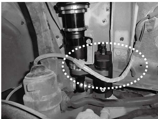
付属スパイラルチューブをタンクと 純正センサーハーネスの干渉する部分に 取り付けて保護してください。
