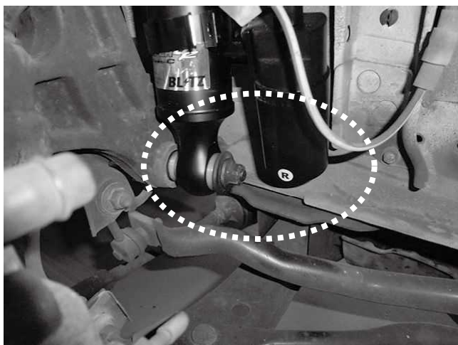
ロアブラケットの取り付けは長い方を ナックル側にして取り付けてください。 ※ナットが取り付けにくい場合はタンク固定ステーを はずして、タンクをずらして作業を行ってください。
