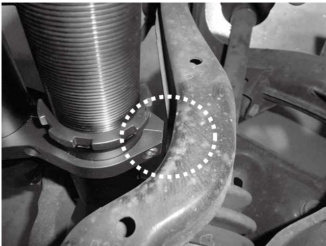
リザーバートank固定ステーと アッパーアームとの干渉に注意してください。
