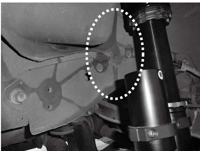
リザーバートankと運転席側インナーフェンダー、 フューエルパイプカバーとの干渉に 注意してください。
