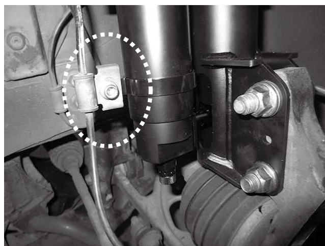
スピードセンサーラインはリザーバータンクに 付属のバンドを使用し取り付けてください。
