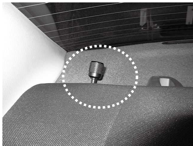
減衰力延長ダイヤル取り付け状態 スピーカーボードに穴をあけて ダイヤルを出しております。
