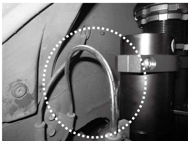
スピードセンサーラインとリザーバータンク 固定ステーとの干渉に注意してください。 ※ステアリングを左右に切った時も確認してください。
