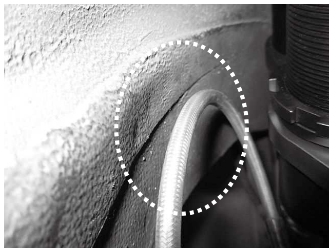
ブレーキラインとボディとの干渉に注意してください。 干渉の可能性がある場合は 同梱スパイラルチューブで保護してください。
