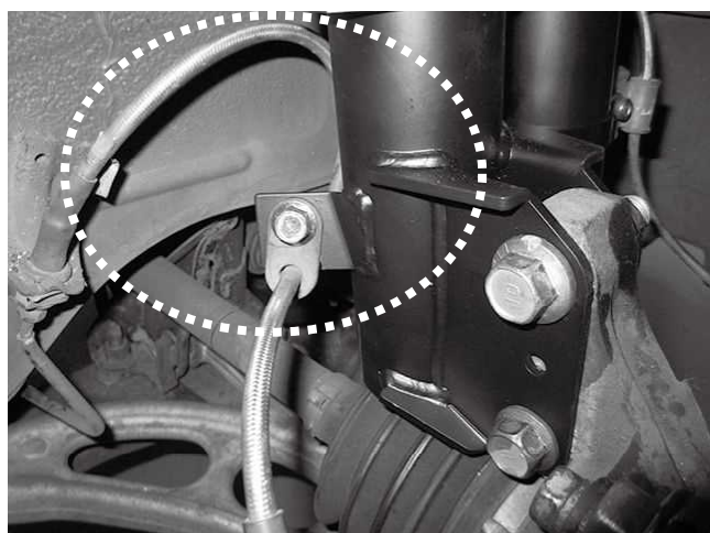
リザーバータンク固定ステーとブレーキライン、 インナーフェンダーとの干渉に注意してください。
