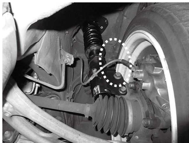
フロント タイヤ・ホイールクリアランス 18×8.0J INSET43 + 25mm 225/40R18装着状態 ※取り付け後クリアランス確認をお願いします。
