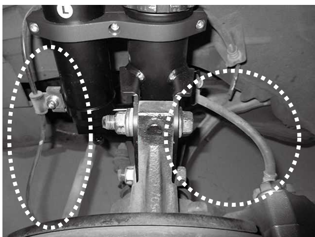
ブレーキライン、スピードセンサーラインの 突っ張りに注意してください。
