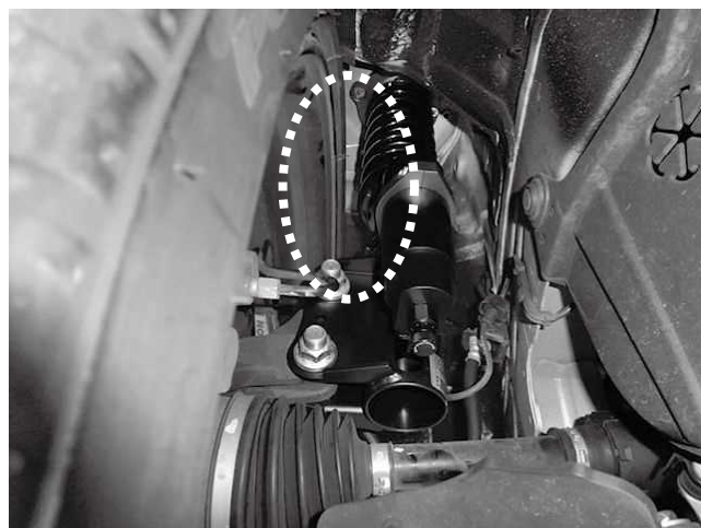
フロント タイヤ・ホイールクリアランス 18×7.5J INSET50 225/40R18装着状態 ※取り付け後クリアランス確認をお願いします。
