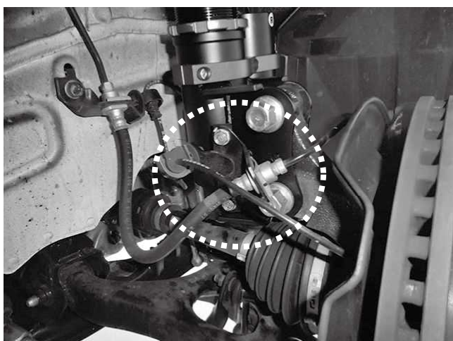
ブレーキラインの固定には純正のステーを使用します。他社品からの付け替えの際はご注意ください。
