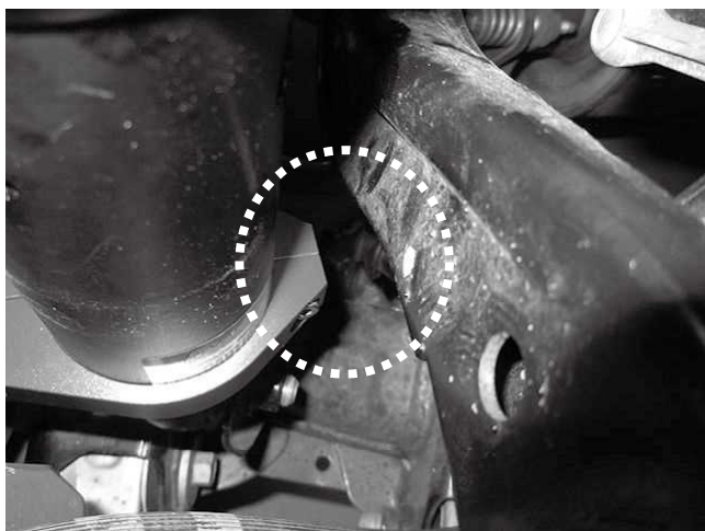
リザーバータンク固定ステーと アッパーアームとの干渉に注意してください。
