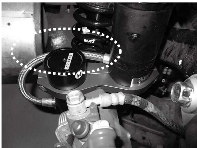
メッシュホースとスプリング、マフラーとの 干渉に注意してください。
