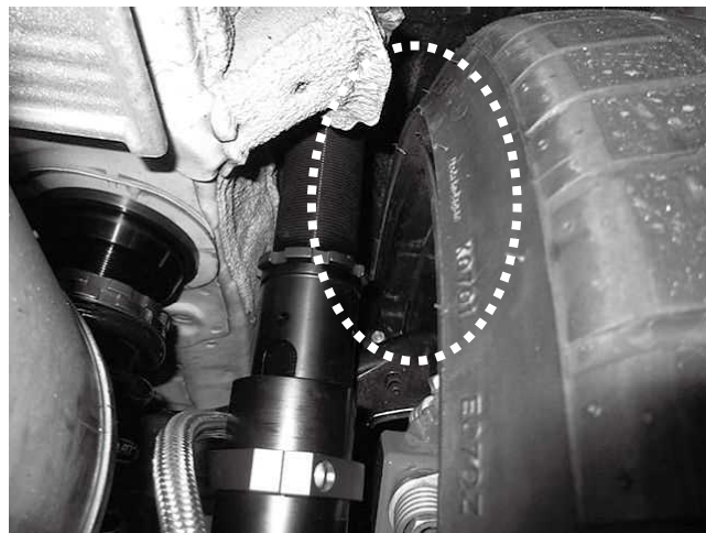
リア タイヤ・ホイールクリアランス 18×8.5J INSET52 225/40R18装着状態 ※取り付け後クリアランス確認をお願いします。
