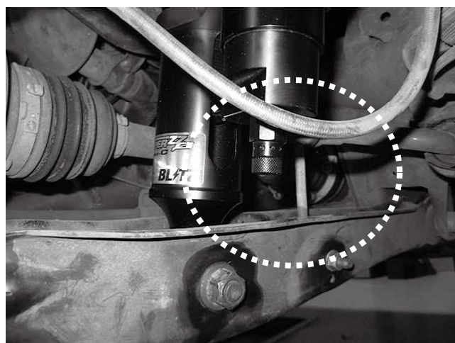
リザーバータンクとブレーキライン、 ロアアームとの干渉に注意してください。
