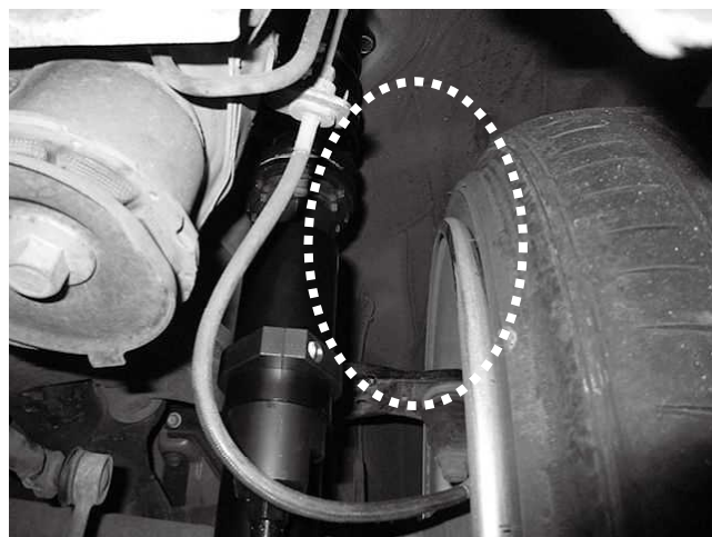
リア タイヤ・ホイールクリアランス 18×9.5J INSET33 225/40R18装着状態 ※取り付け後クリアランス確認をお願いします。
