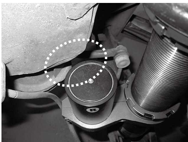
リザーバータンク(固定ステア)と インナーフェンダーとの干渉に注意してください。
