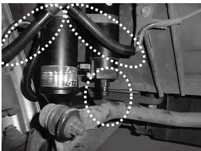
リザーバータンクとスタビライザーとの 干渉に注意してください。 ブレーキライン、スピードセンサーラインは 同梱スパイラルチューブで保護してください。
