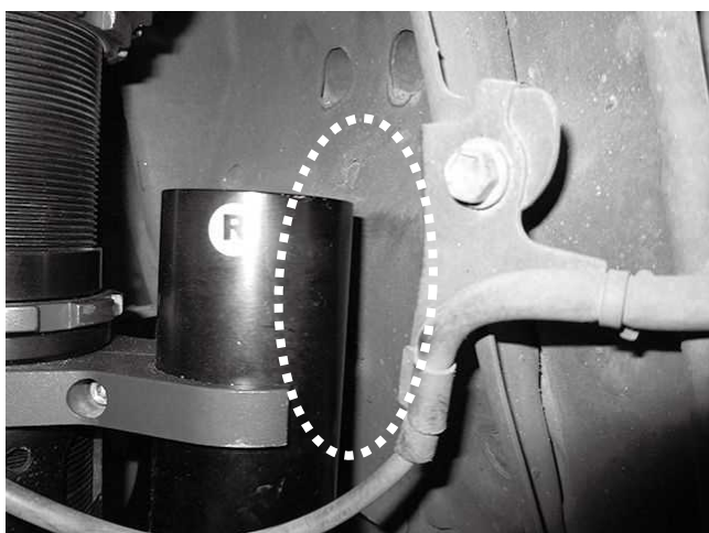
リザーバータンクとボディとの 干渉に注意してください。
