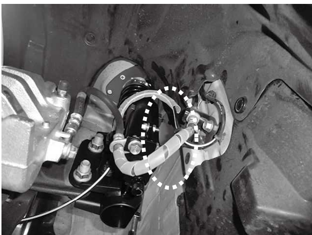
リザーバータンク・スタビリンクと インナーフェンダーとの干渉に注意してください。 ※ステアリングを切ったときに干渉しないかも確認してください。
