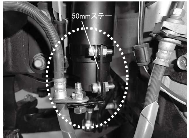
付属ナット、ステー、純正ボルトを使用してブレーキラインを固定して ください。基準車高では同梱している約50mmステーを使用してください。 車高を上げる、ホイールが小径の場合などでブレーキラインと ホイール内側が干渉する際は約90mmのステーを使用してください。
