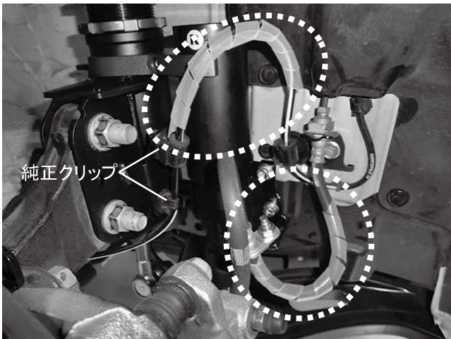
付属品スパイラルチューブを上写真の 位置に取り付けてください。ABSセンサーハーネス 固定は純正クリップを使用してください。
