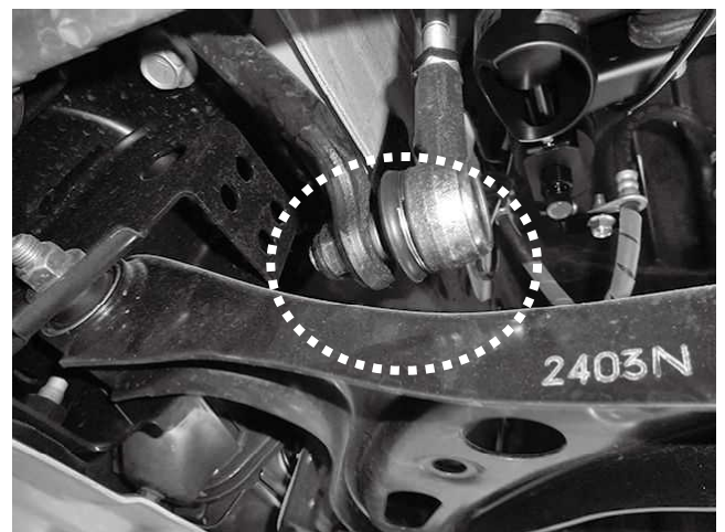
スタビリンクとロアアームとの干渉に 注意してください。干渉する場合は、 スタビリンクの長さを調整してください。
