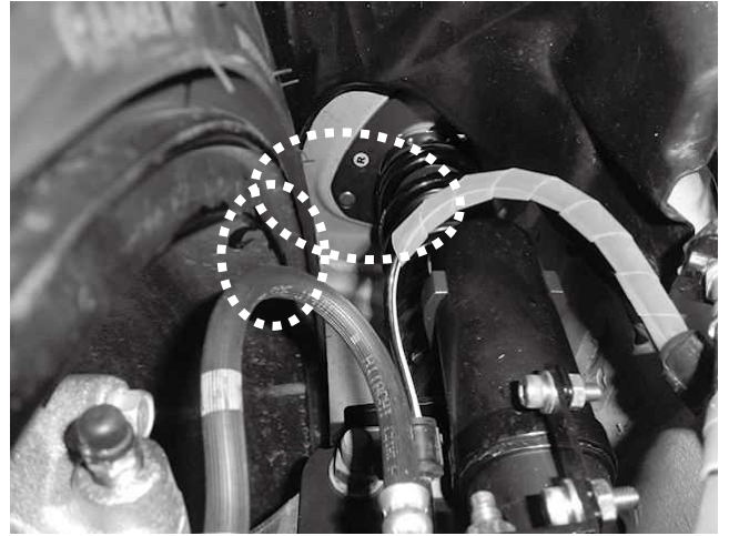
フロント タイヤ・ホイールクリアランス 純正ホイール(17インチ)・タイヤ装着状態 ※取り付け後クリアランス確認をお願いします。
