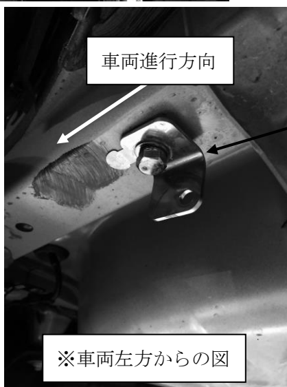
専用ステー ※M10×35 を使用
