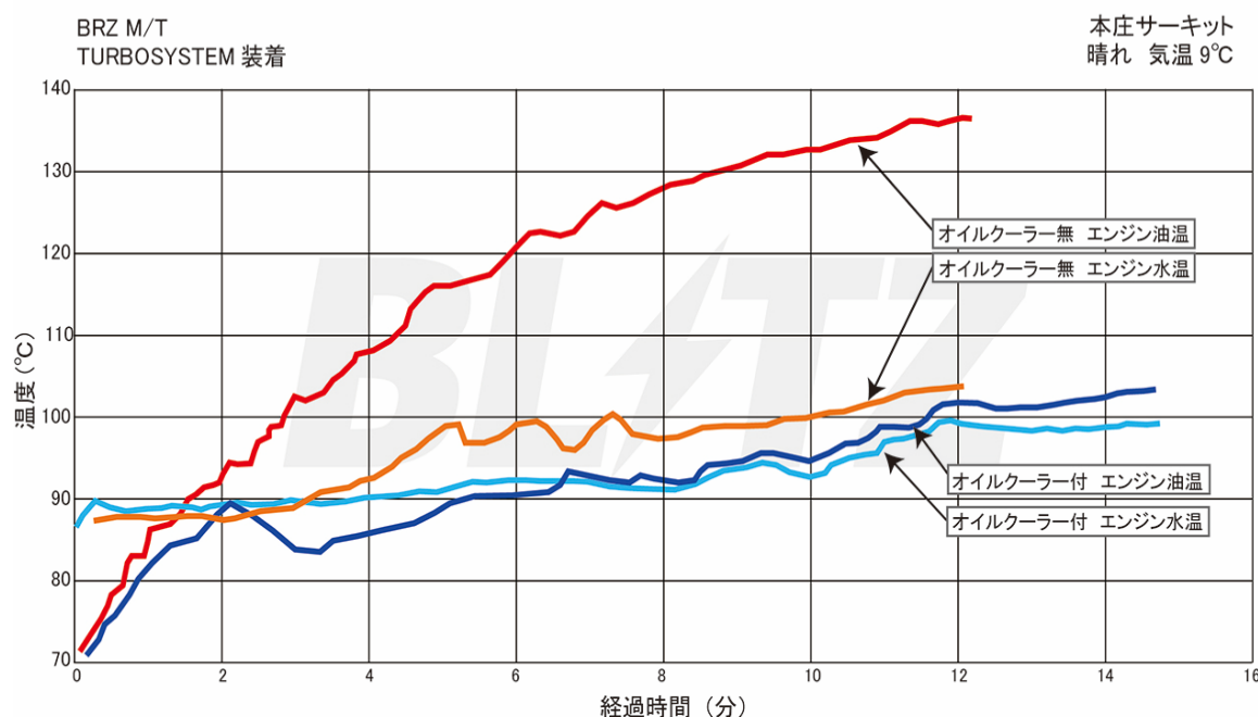
エンジン油温 / 水温 経過比較グラフ
