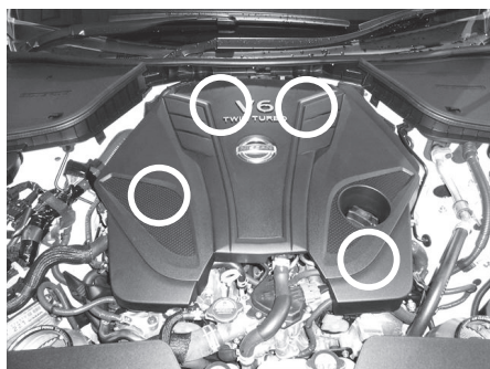
スカイライン エンジンカバー グロメット 4カ所（丸部）
