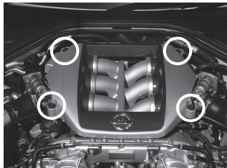
エンジンカバー ボルト4カ所（丸部）
