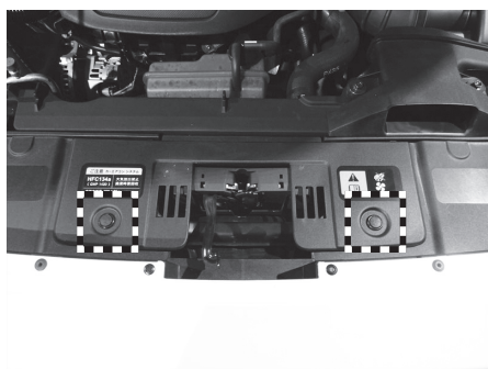
フロントバンパー (クリップ × 2)
