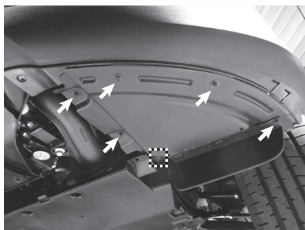
インナーフェンダーフロント側 (クリップ × 1、ビス × 5)
