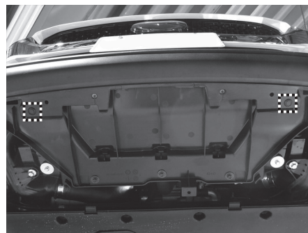
フロントバンパー アンダー側 (クリップ × 2)
