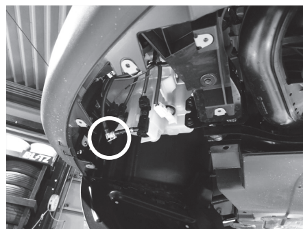
ウォッシャーホース (ホースコネクタ)
