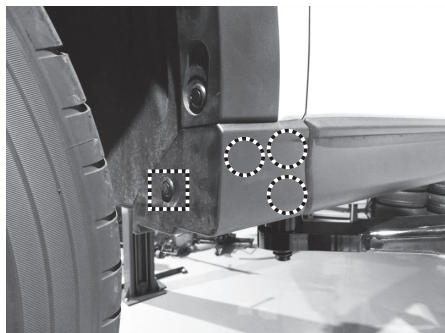
オーバーフェンダーロア (クリップ × 1、ツメ × 3)
