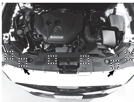
ライトコネクタ (クリップ × 6、ボルト × 4)
