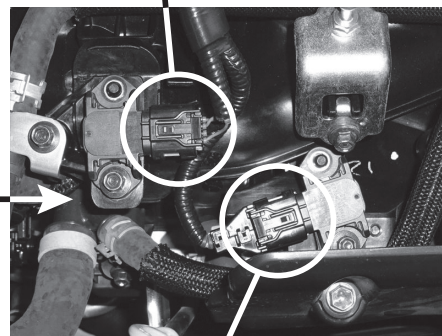
こちらの圧力センサーに接続
