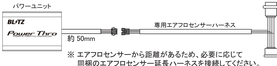
パワーユニット ハーネス
