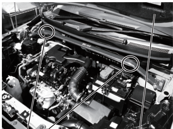
クリアランス確認箇所 タワーバーシャフトとボンネットインシュレーターとの クリアランス約11mm
