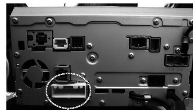
アクセサリ電源の取れる20ピンコネクター
