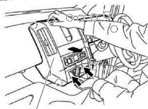
クラスターリッド かん合 ↑ネジ
