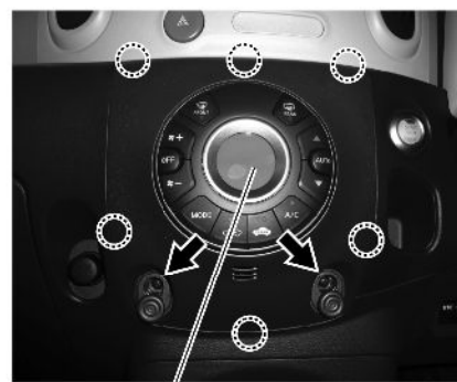
フロントコントローラー かん合 ↑ネジ
