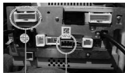
6ピンコネクター アクセサリ電源の取れる20ピンコネクター
