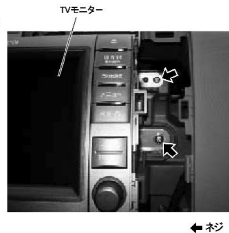
インストルメントクラスタフィニッシュパネルCTR
