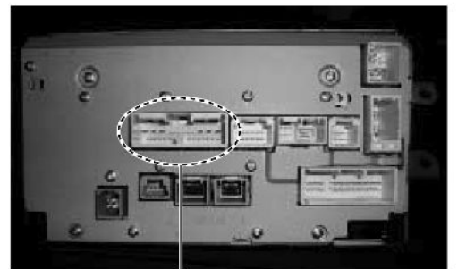
26ピンコネクター
