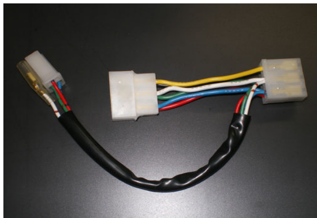
TURBO TIMER HARNESS(イメージ写真)
