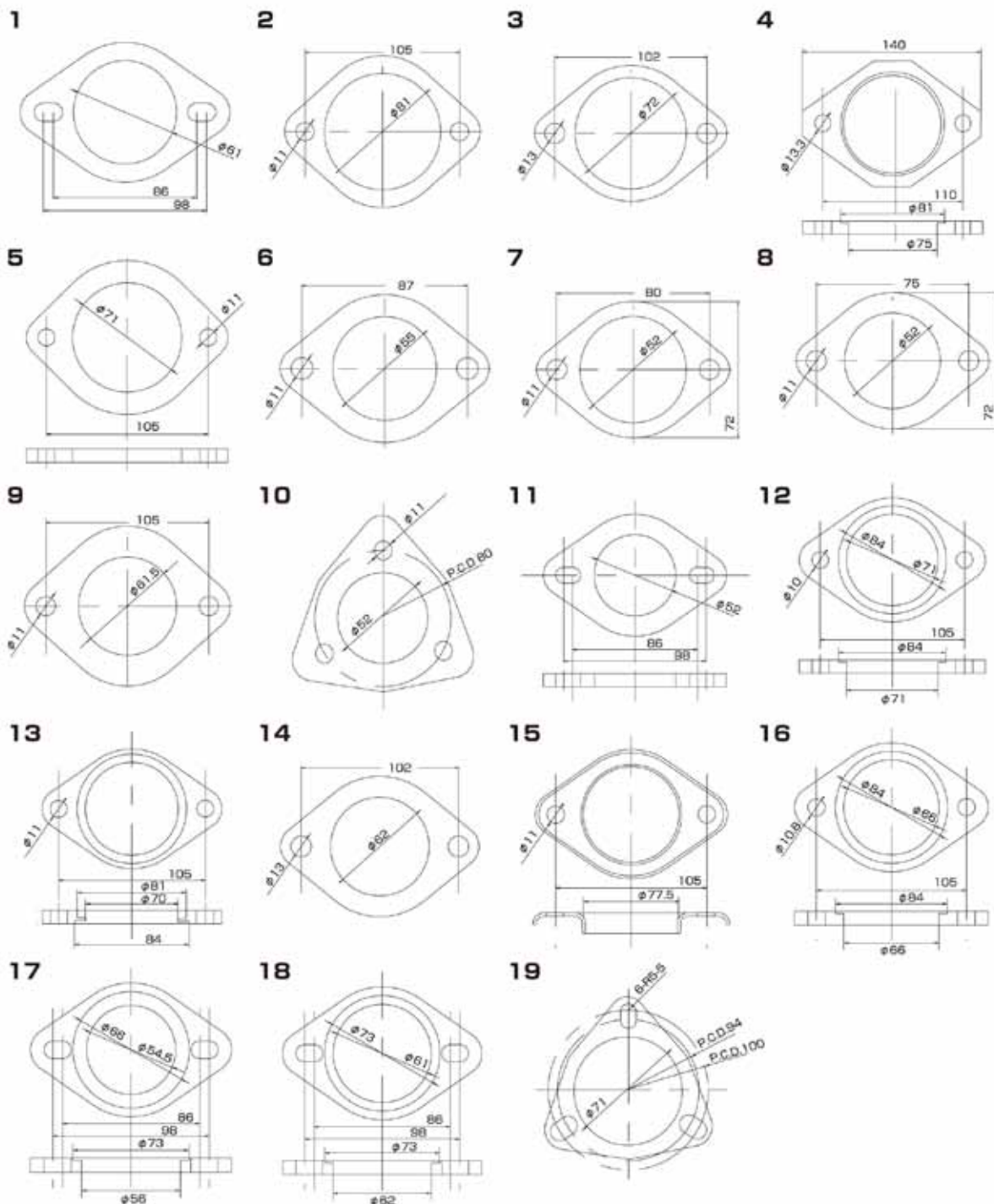
マフラーフランジ(スチール)&適合ガスケット
