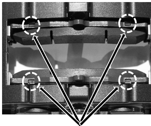
ブレーキパッド上部の溝
