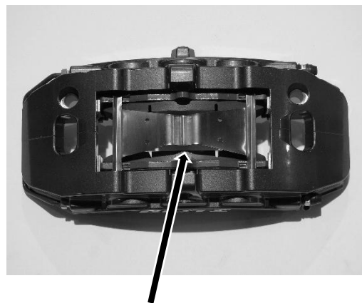
パッドスプリング
