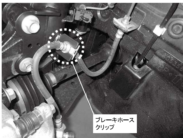
ブレーキホースクリップ取り付け
