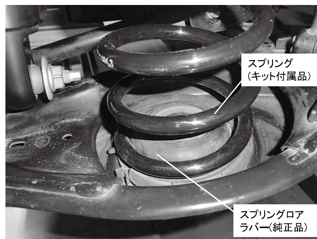
リアスプリングロアアーム側取り付け状態
