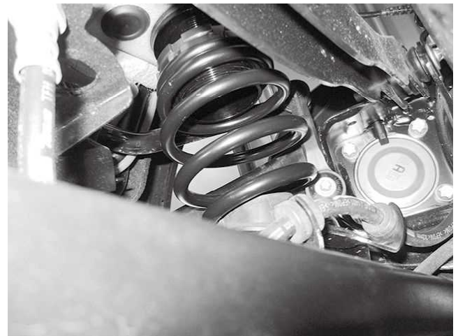
リアスプリング車両取り付け状態 上写真を参照し、スプリングを車両に 取り付けてください
