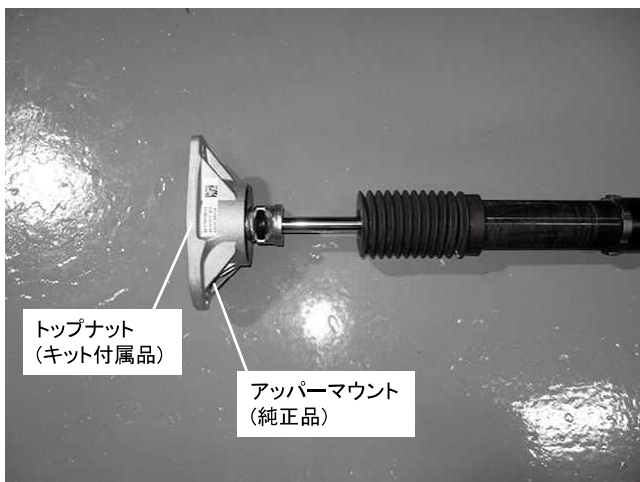
リアショックアッパーマウント取り付け状態 ※純正ショックよりアッパーマウントを取り外し キット付属トップナットを使用して組みつけてください
