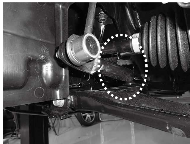
スタビライザーとドライブシャフト、ロアアームと 干渉がないか確認してください
