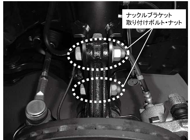
ナックルブラケット取り付けボルト・ナット 2カ所締め付け 締め付けトルク: 108N・m(11.0kgf・m)
