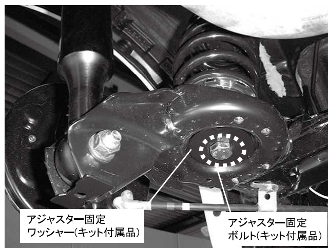
リアアジャスター固定ボルト・ナット
