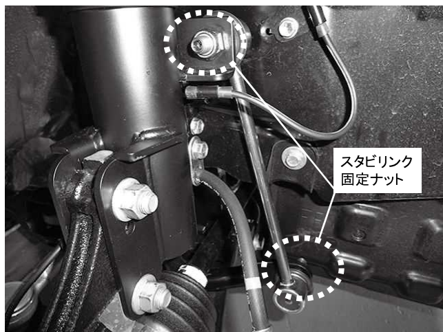
スタビリンク固定ナット 2カ所締め付け 締め付けトルク: 48N・m(4.9kgf・m)
